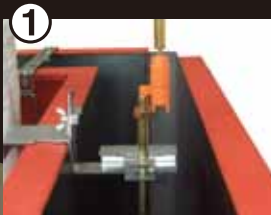
① アンカーアイに固定したアンカーボルトの 高さ位置を決める
