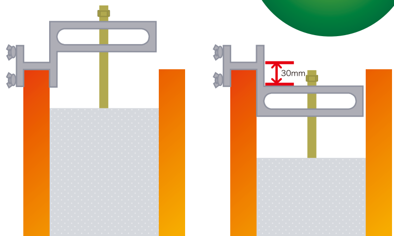
アンカーボルトが型枠天端より下がる場合(-30mmまで)、 右図の取付で施工可能。
